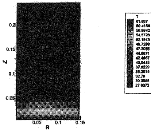
شکل (۱۱ - ب) کانتور تغییرات دمای ذرات در بستر فشرده t = 100 \text{ sec} .
