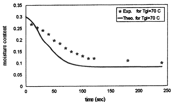
شکل (۱۵) تغییرات محتوی رطوبت تئوری - تجربی ذرات در بستر شناور.
