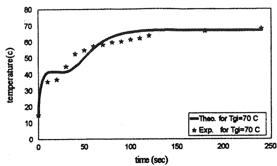
شکل (۱۴) تغییرات دمای تئوری - تجربی گاز داخل بستر شناور.
