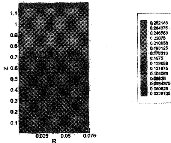
شکل (۱۲ - الف) کانطور تغییرات رطوبت ذرات در بستر شناور t = 100 sec
