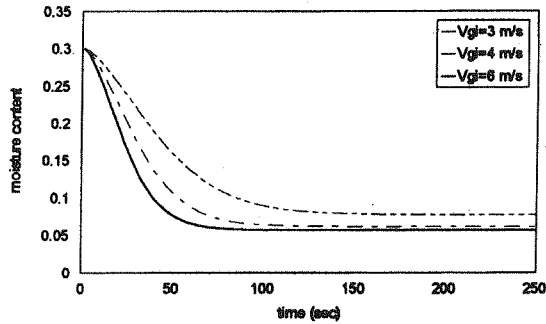
شکل (۹) تغییرات محتوی رطوبت ذرات در بستر شناور.
