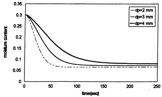
شکل (۷) تغییرات محتوی رطوبت ذرات در بستر شناور.
