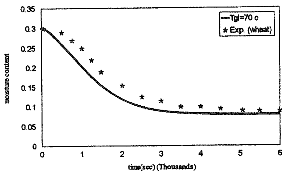
شکل (۱۶) تغییرات محتوی رطوبت تئوری - تجربی ذرات در بستر فشرده.
