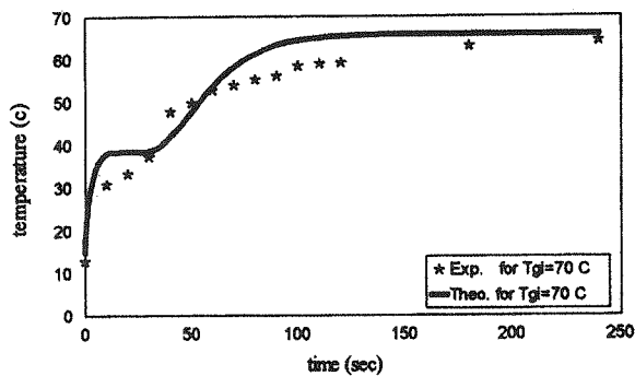
شکل (۱۳) تغییرات دمای تئوری - تجربی ذرات گندم در بستر شناور.
