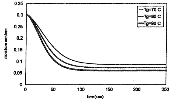
شکل (۵) تغییرات محتوی رطوبت ذرات در بستر شناور.
