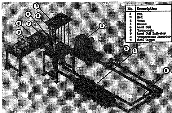
شکل (۳) مدل آزمایشگاهی دستگاه بستر شناور.
