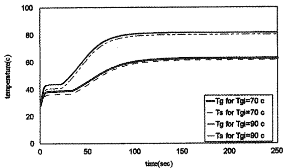
شکل (۴) تغییرات دمای گاز و ذرات در بستر شناور.
