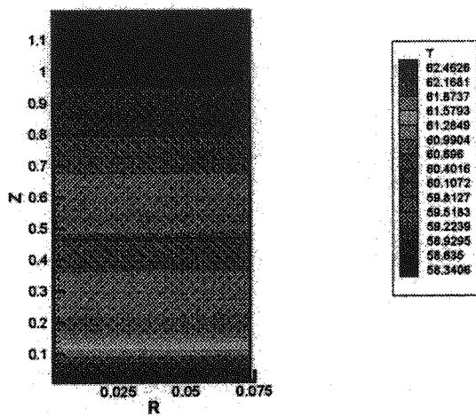
شکل (۱۲ - ب) کانطور تغییرات دمای ذرات در بستر شناور t = 100 sec
