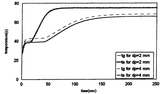
شکل (۶) تغییرات دمای گاز و ذرات در بستر شناور.
